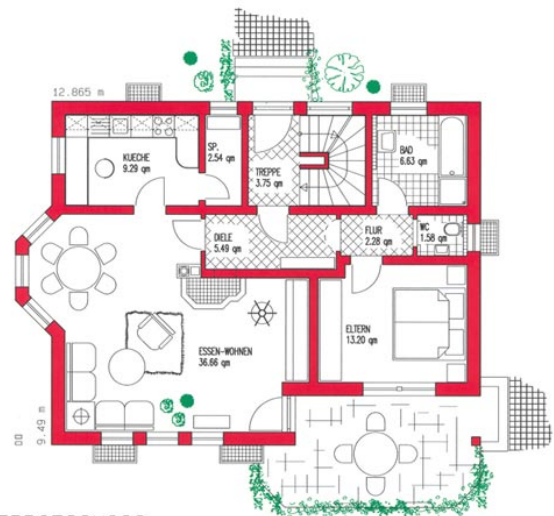
ERDGESCHOSS HAUS BAMBERG
